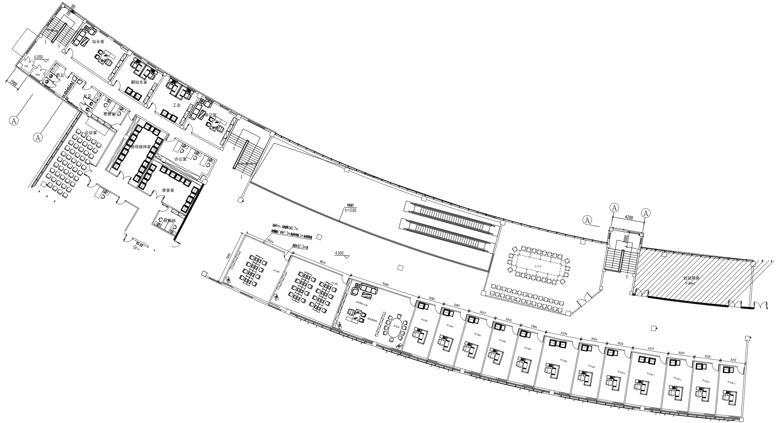
二层平面布置图 1:250
